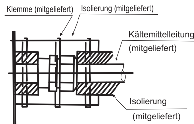
Rohrleitungsisolierungsvorgang
