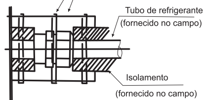
Procedimento de isolamento de tubulações
