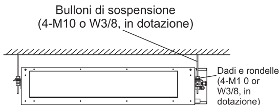
Fig. 3.4 Installazione dell'unità interna
