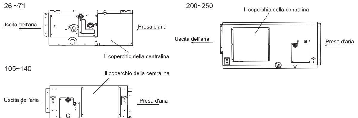
Fig.6.1 Rimuovere le viti sulla centralina.
