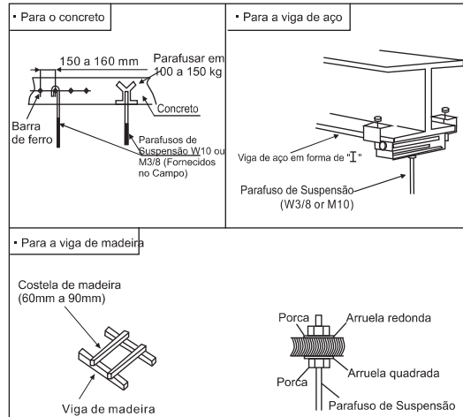
Fig. 3.5 Fixação dos parafusos de suspensão
