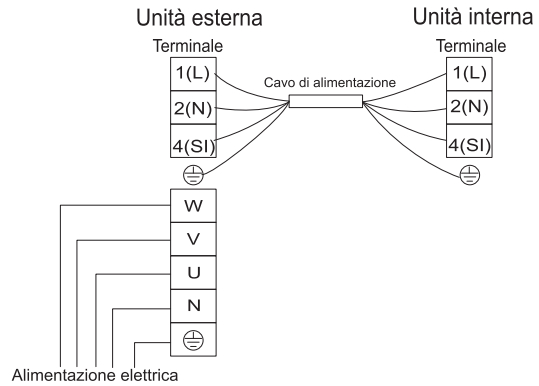
Serie trifase
