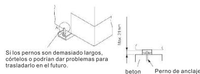
Fig. 2 Instalación de los pernos de anclaje
