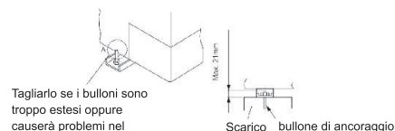
Fig.2 L'installazione dei bulloni di ancoraggio
