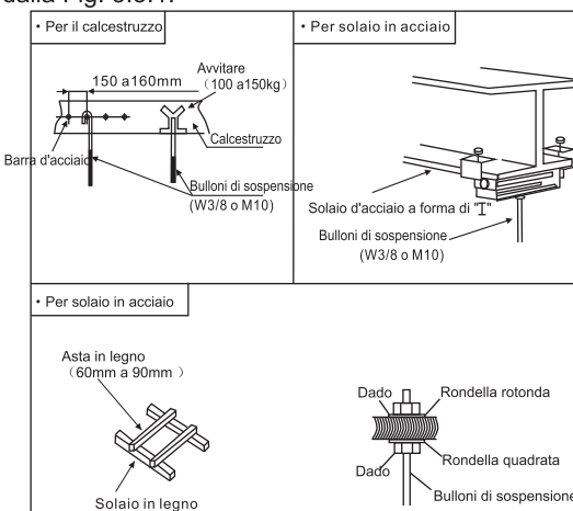
Fig. 3.3.1. Fissaggio dei bulloni di sospensione
