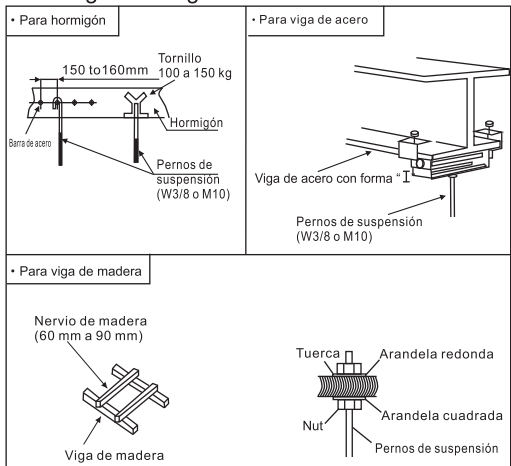
Fig. 3.3.1 Fijar los pernos de suspensión 3.3.2 Posición de los pernos de suspensión y las tuberías
