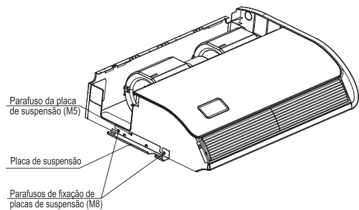
Figuras. 3.3.6 Parafusos e porcas de suspensão
