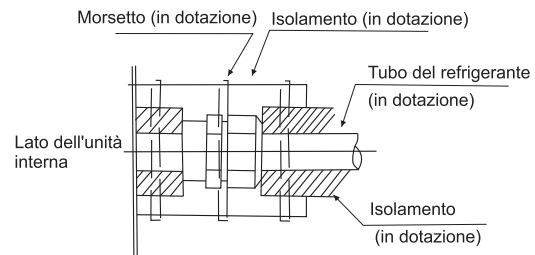
Fig. 4.5 Procedura di isolamento dei tubi
