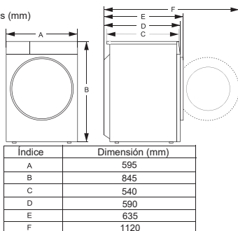
Dimensiones (mm)
