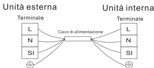
Schema del cablaggio elettrico
