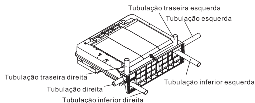
Fig. 4.1 As posições de conexão do tubo
