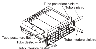
Fig. 4.1 La posizione di connessione del tubo
