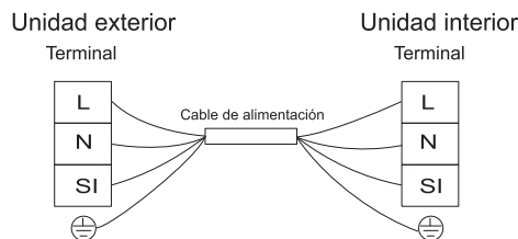
Diagrama de cableado eléctrico
