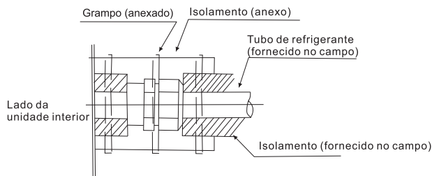
Fig. 4.4 Procedimento de isolamento da tubagem
