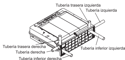
Fig. 4.1 Posiciones de conexión de la tubería
