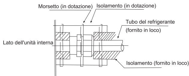
Fig 4.4 Procedura di isolamento dei tubi
