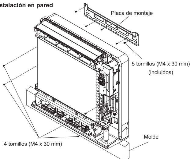
Instalación en pared
