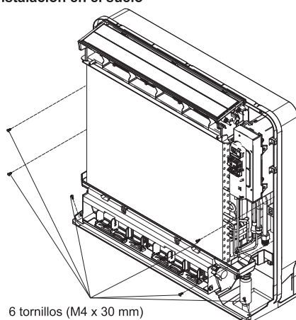
Instalación en el suelo
